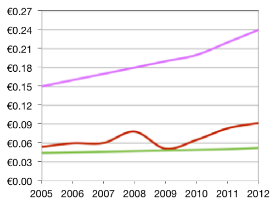
Energieprijsevolutie 2005-2012 (euro/kWh)
